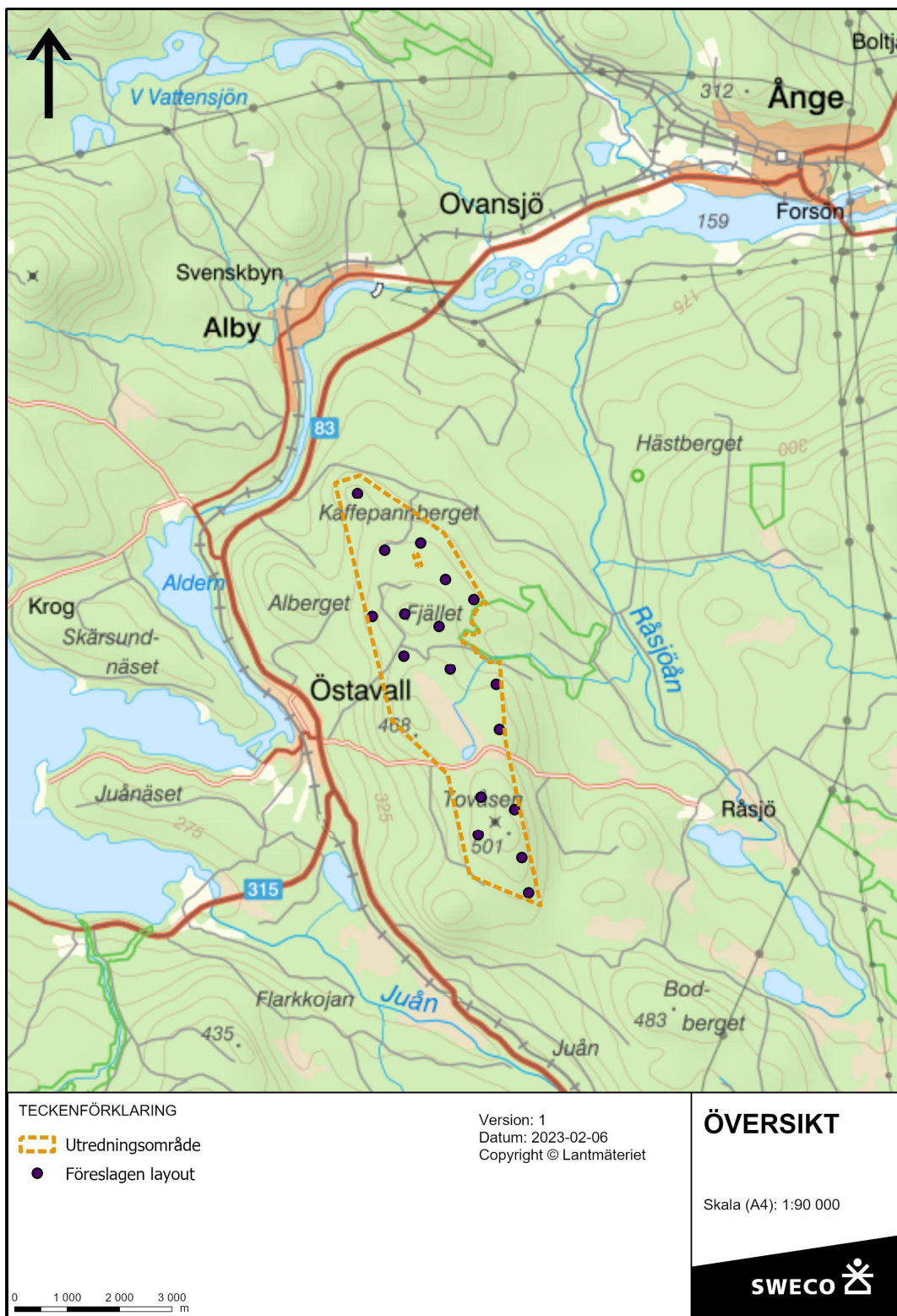
Figur 1. Föreslagen layout för vindpark Östavall.
